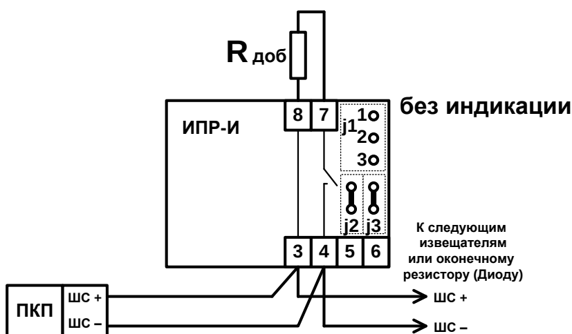
Рис 3. Включение ИПР-И и его эквивалентные схемы в режиме НР-контакта в шлейфе сигнализации с токопотребляющими извещателями (имитация дымового пожарного извещателя). Величина R_{доб} устанавливается в соответствии с техническим описанием ПКП.
